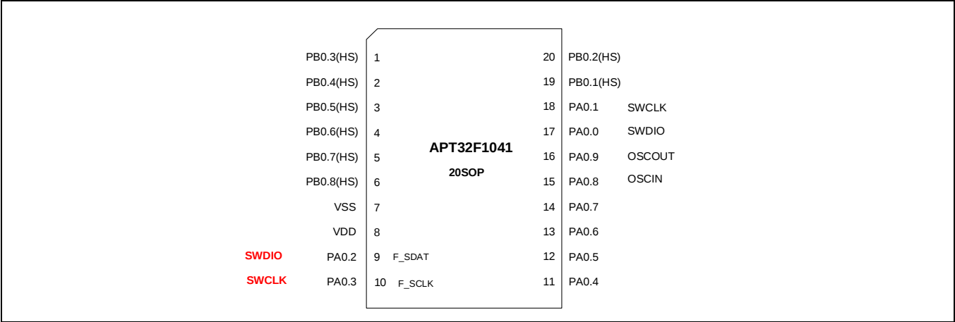
Figure 2-3 管脚定义图(SOP20)
